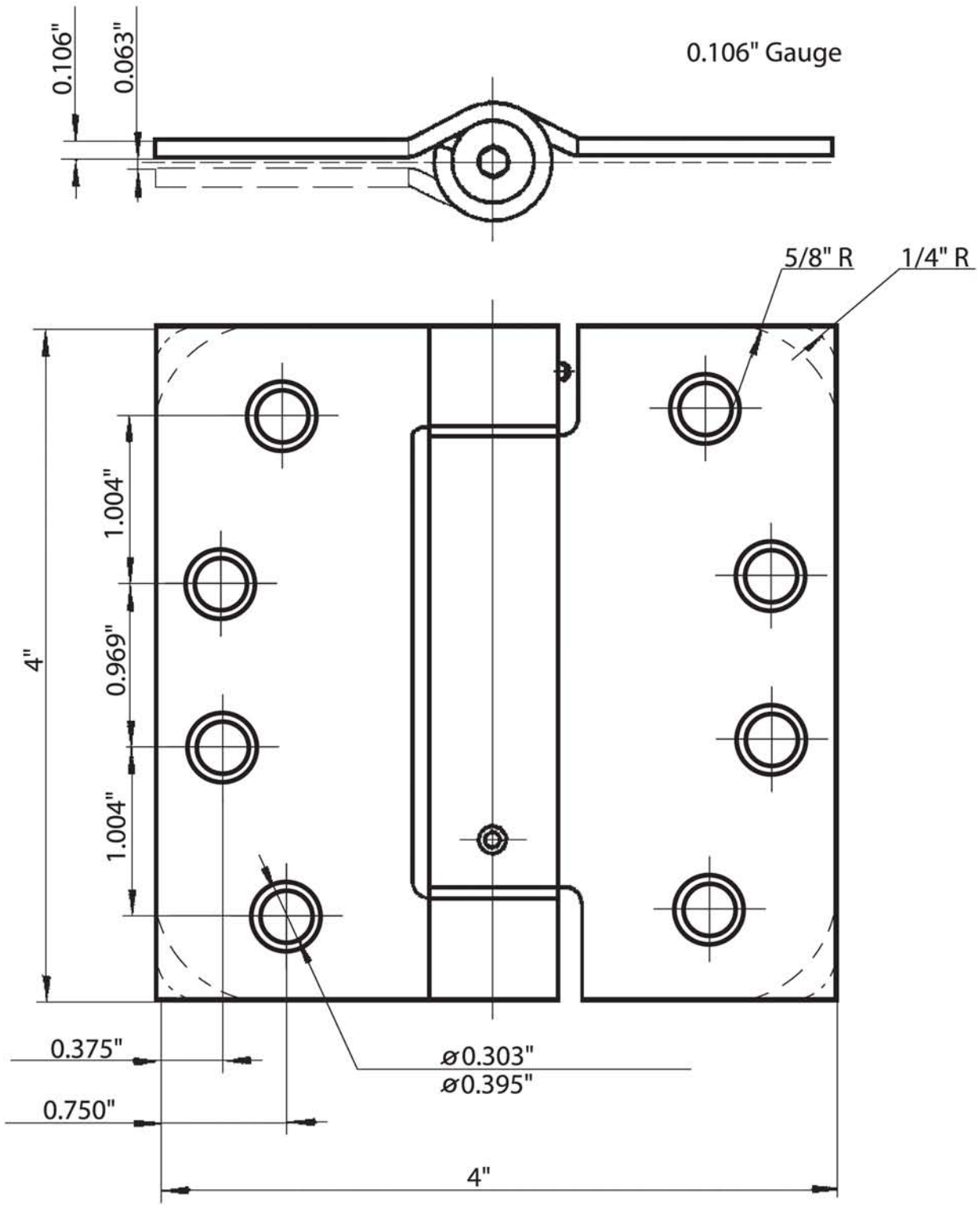
SP410 420 450 Spring Hinge
